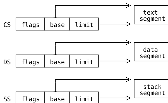
Figura 3: Registros de segmentos.
